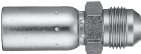
3/8" x 7/8-14 (-10) Male JIC 37° Flare
